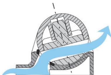
Drehverschluss geöffnet
