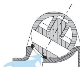
Drehverschluss geschlossen
